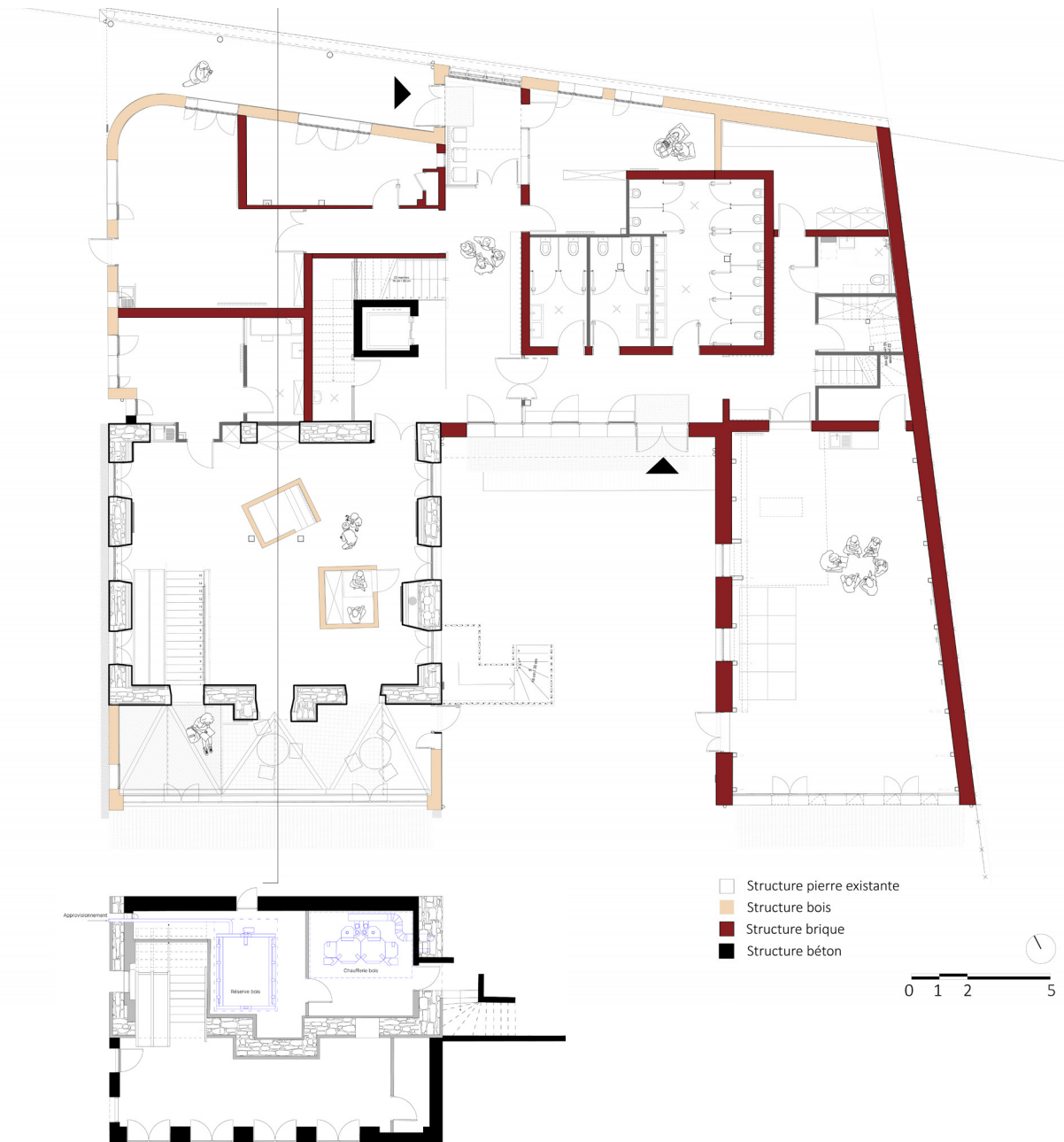
Plan RDC
