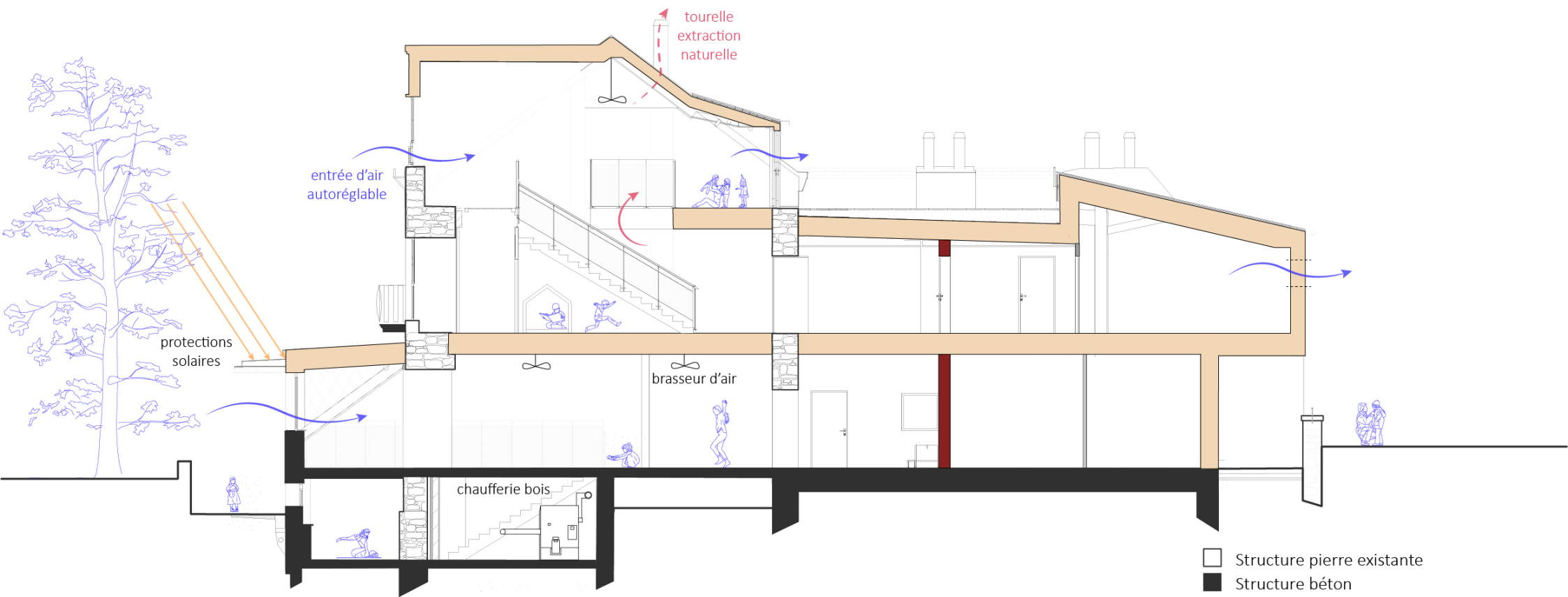
Coupe transversale bioclimatique
