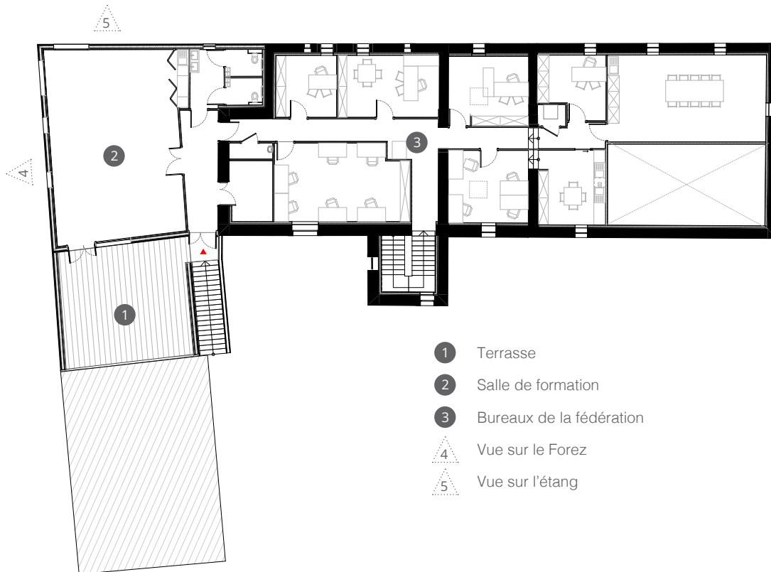
Plan du R+1
